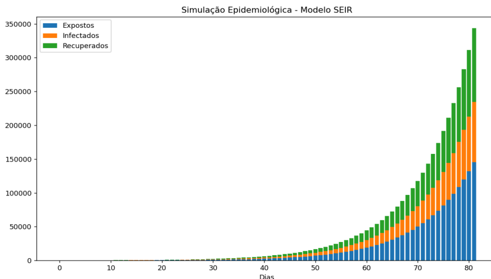
Figura 1 – Evolução das classes epidemiológicas do modelo SEIR.
